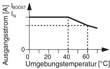
Bild 14 Temperaturverhalten
