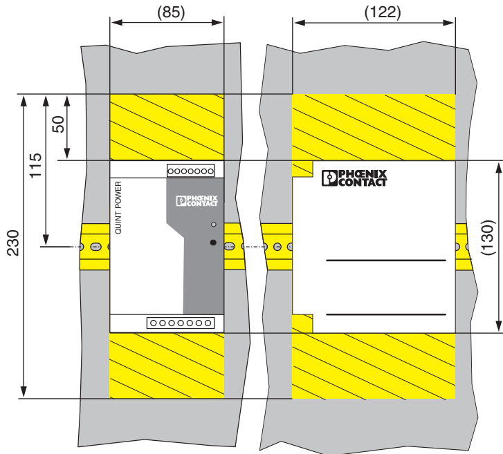
Bild 4 Einbaulage (Maße in mm)
