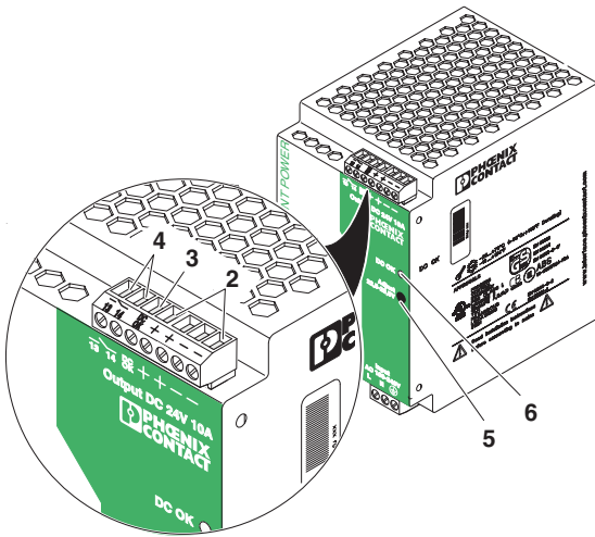
Bild 9 Ausgang
