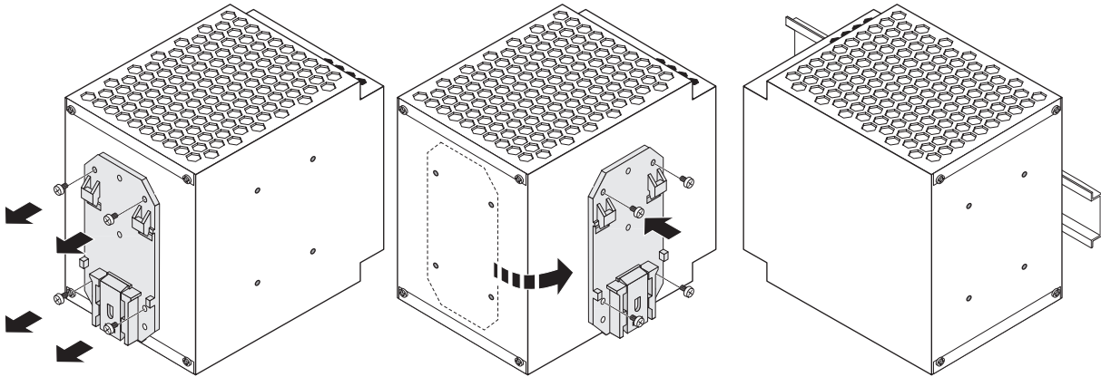
Bild 6 Flache Einbaulage
