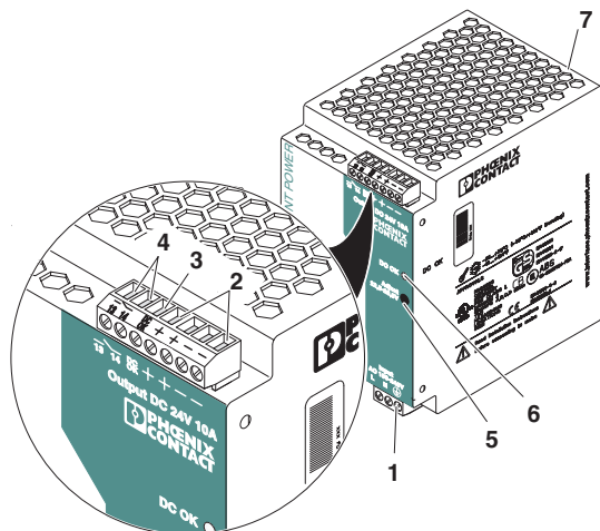
Bild 1 Bedienelemente
